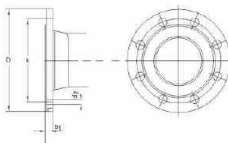
Flange
