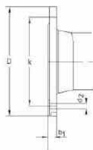
Flange
